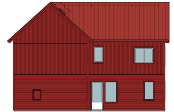
LÄGENHET 7H FASAD MOT SYDVÄST
